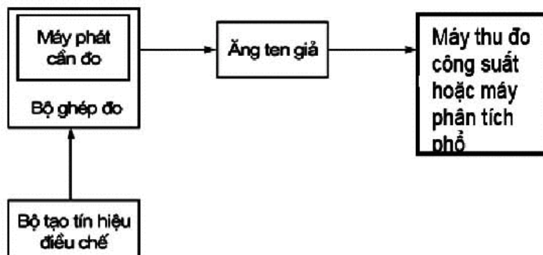
Hình 5 - Sơ đồ đo công suất kênh lân cận và kênh khác
