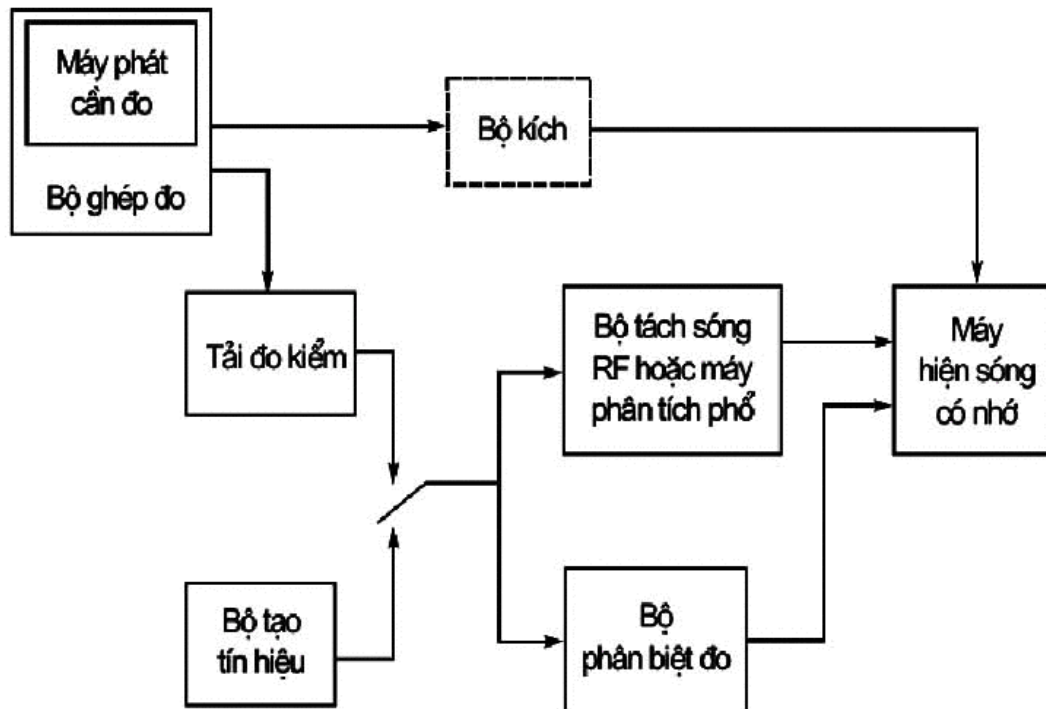
Hình 8 - Sơ đồ đo đáp ứng quá độ của công suất máy phát và tần số, bao gồm thời gian kích hoạt và thời gian khử hoạt máy phát
