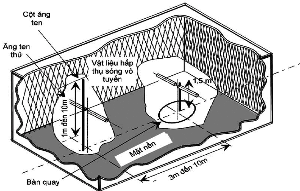
Hình A.2 - Buồng đo không phản xạ có mặt phẳng tiếp đất
