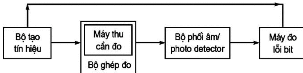
Hình 15 - Sơ đồ đo độ nhạy với luồng bit liên tục ở điều kiện đo tới hạn
