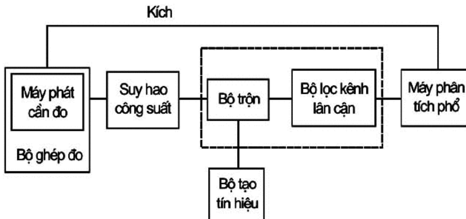
Hình 13 - Sơ đồ bố trí thiết bị đo công suất quá độ kênh lân cận
