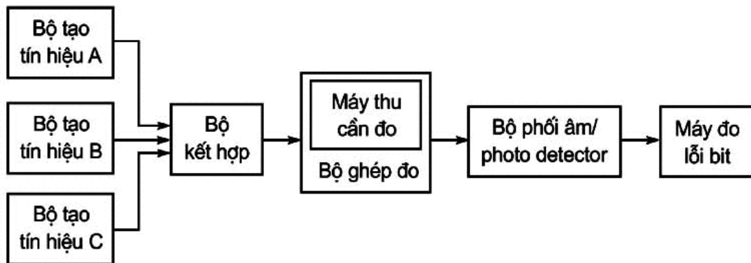
Hình 25 - Sơ đồ đo triệt đáp ứng xuyên điều chế đối với luồng bit liên tục
