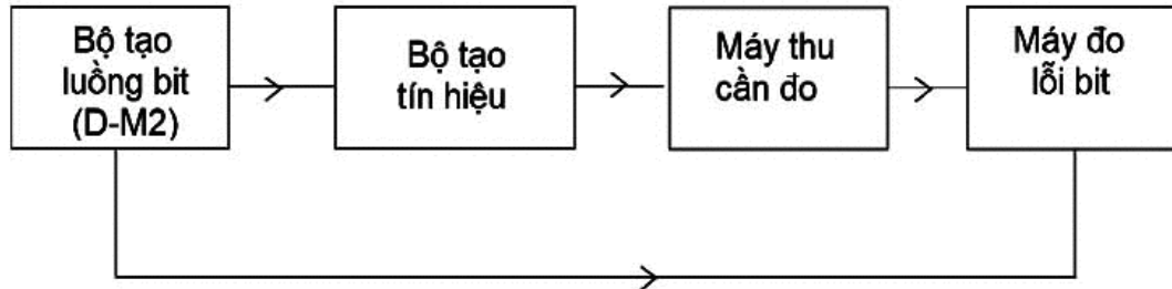
Hình 18 - Phương pháp đo hiệu suất lỗi đối với luồng bit liên tục
