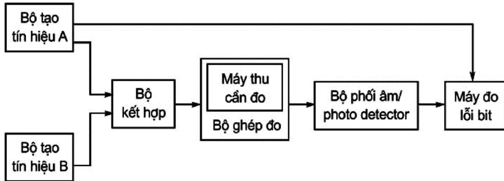
Hình 22 - Sơ đồ đo độ chọn lọc kênh lân cận đối với luồng bit liên tục
