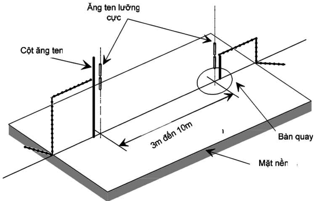
Hình A.3 - Vị trí đo ngoài trời
