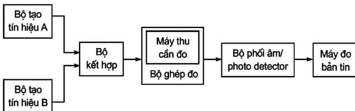
Hình 23 - Sơ đồ đo độ chọn lọc kênh lân cận đối với các bản tin
