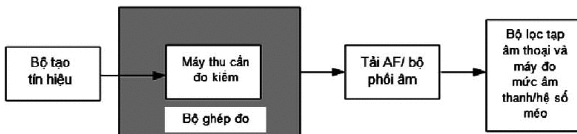
Hình A.6 - Sơ đồ đo để hiệu chỉnh
