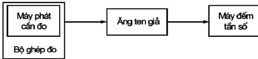
Hình 1 - Sơ đồ đo sai số tần số
