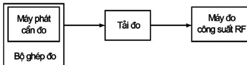
Hình 4 - Sơ đồ đo công suất bức xạ hiệu dụng trung bình và cực đại trong điều kiện đo tới hạn
