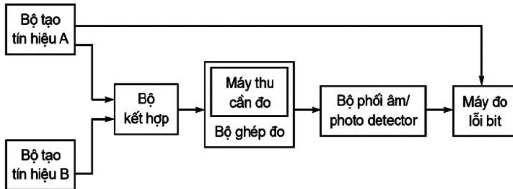
Hình 20 - Sơ đồ đo triệt nhiễu đồng kênh đối với luồng bit liên tục
