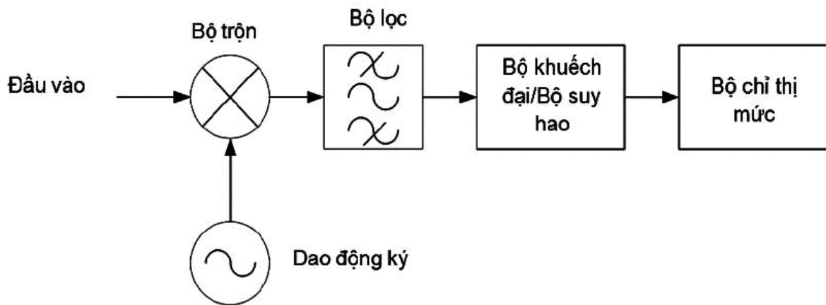
Hình B.1 - Máy thu đo công suất
