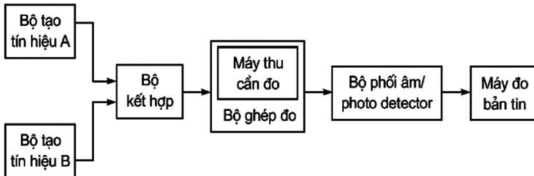
Hình 21 - Sơ đồ đo triệt nhiễu đồng kênh đối với các bản tin
