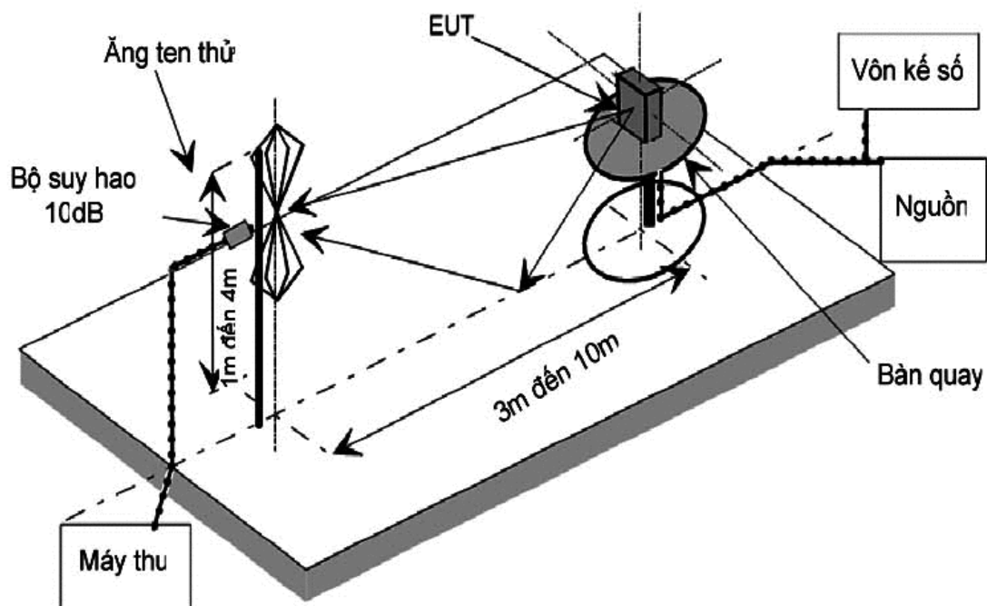
Hình A.4 - Bố trí phép đo tại vị trí đo có mặt phẳng tiếp đất (Thiết lập OATS cho đo phát xạ giả)
