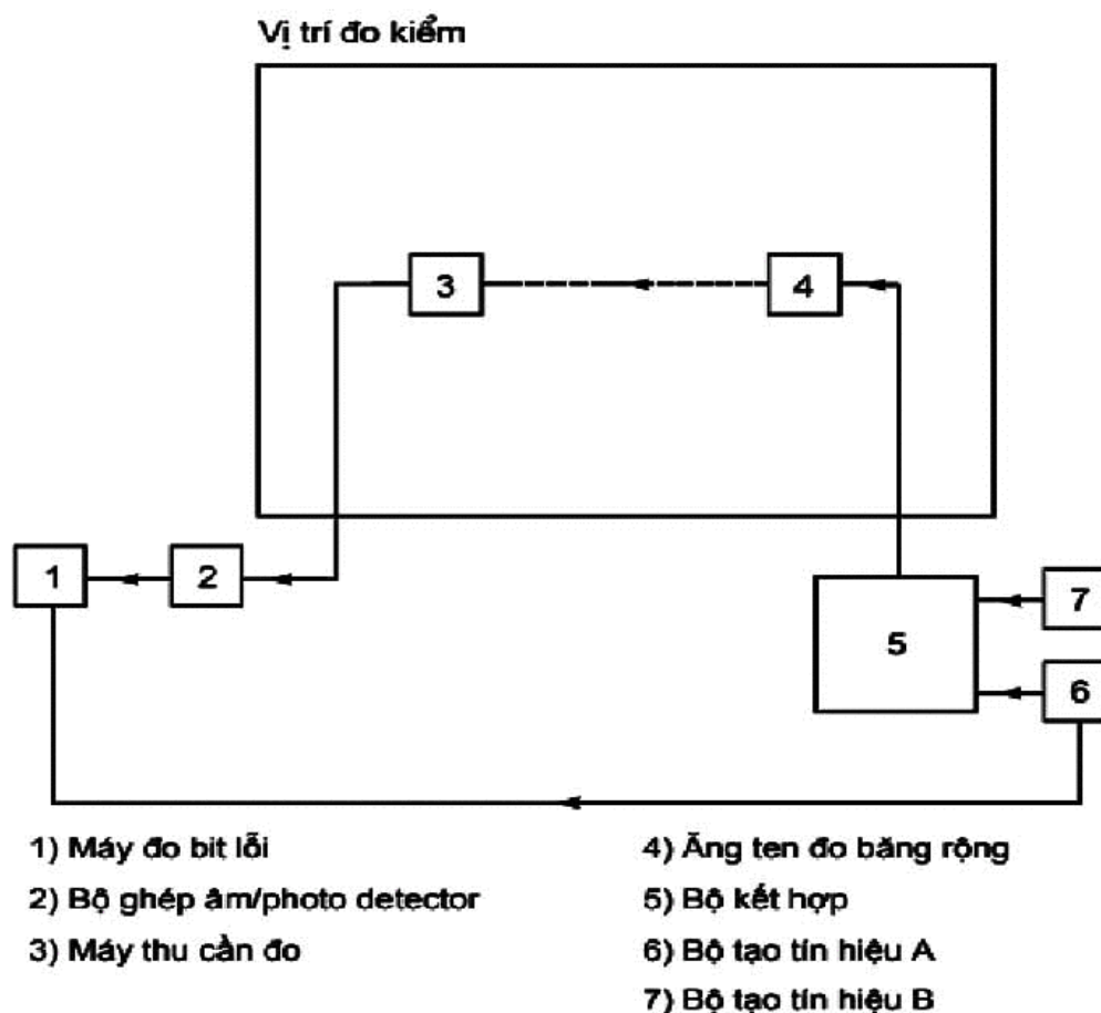
Hình 27 - Sơ đồ đo đặc tính chặn đối với các luồng bit liên tục
