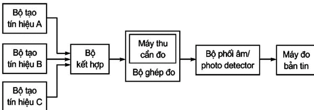
Hình 26 - Sơ đồ đo triệt đáp ứng xuyên điều chế đối với các bản tin
