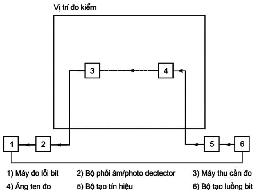
Hình 14 - Sơ đồ đo độ nhạy với luồng bit liên tục ở điều kiện đo bình thường
