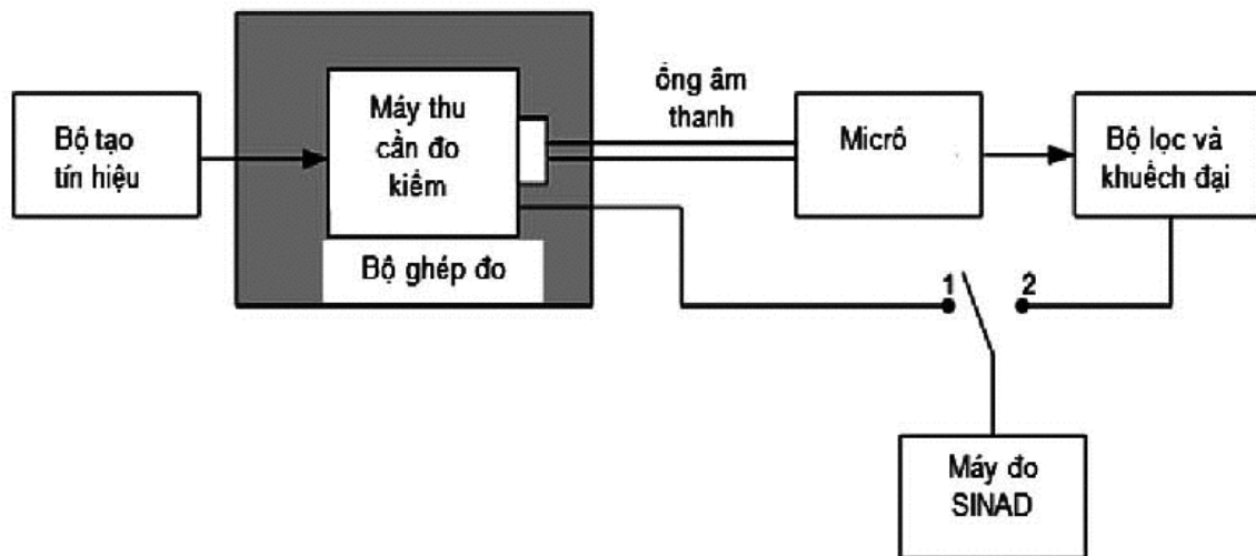
Hình A.5 - Sơ đồ đo để hiệu chỉnh
