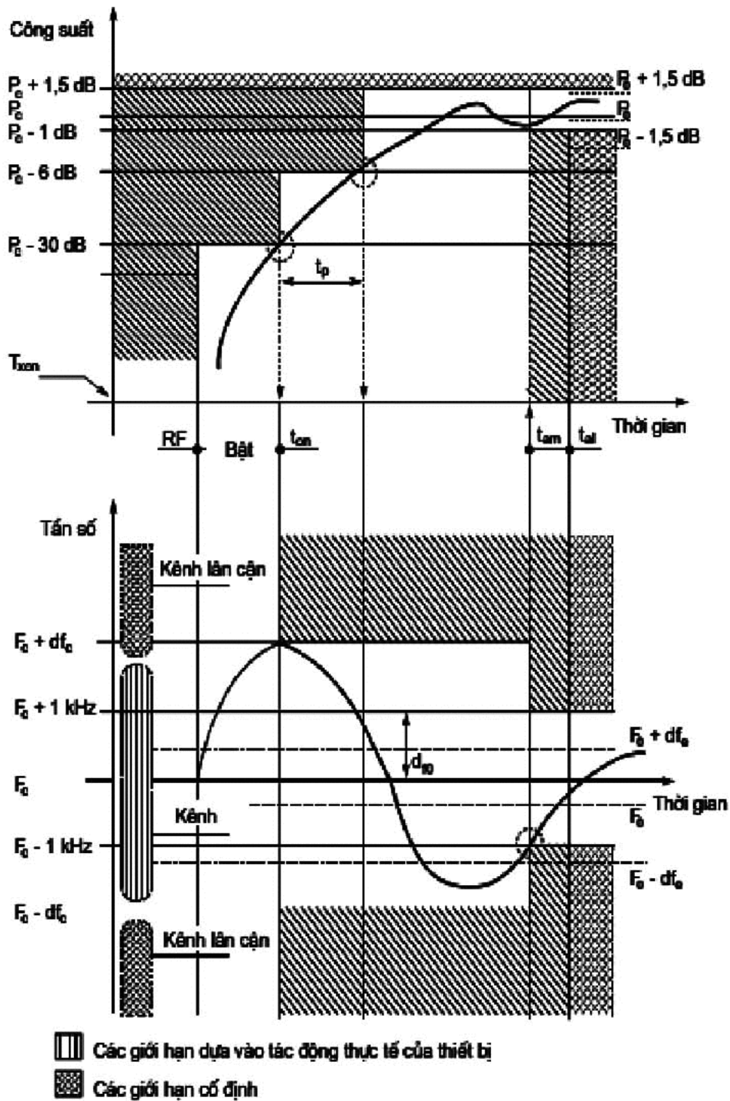
Hình 10 - Thời gian kích hoạt máy phát và tác động quá độ trong khi bật máy (Tác động quá độ của tần số khi bật máy)
