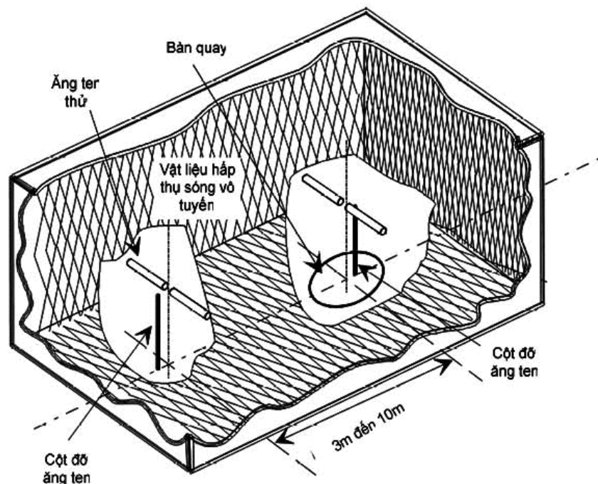
Hình A.1 - Buồng đo không phản xạ
