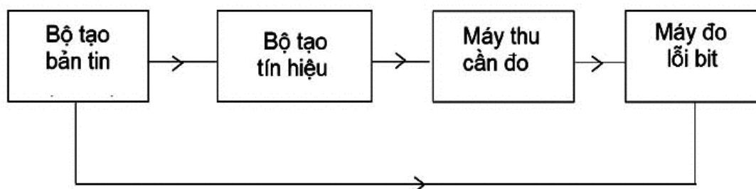
Hình 19 - Phương pháp đo hiệu suất lỗi đối với các bản tin
