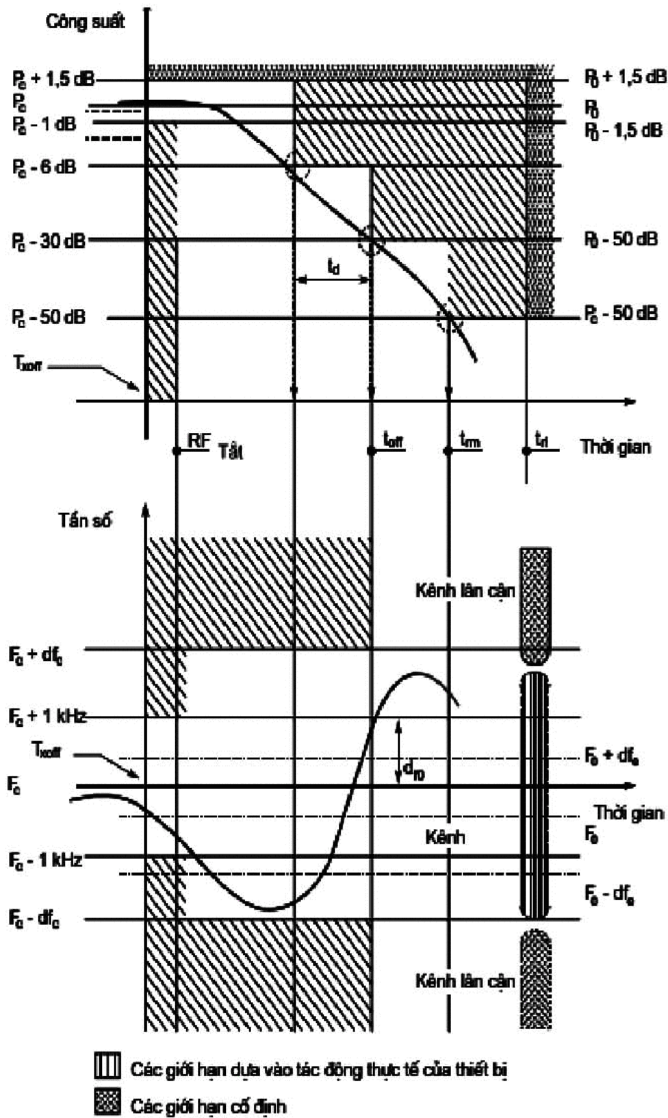
Hình 11 - Thời gian khử hoạt máy phát và tác động quá độ trong khi tắt máy
