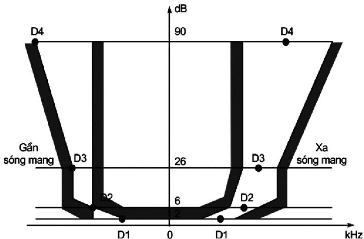
Hình B.2 - Bộ lọc IF
