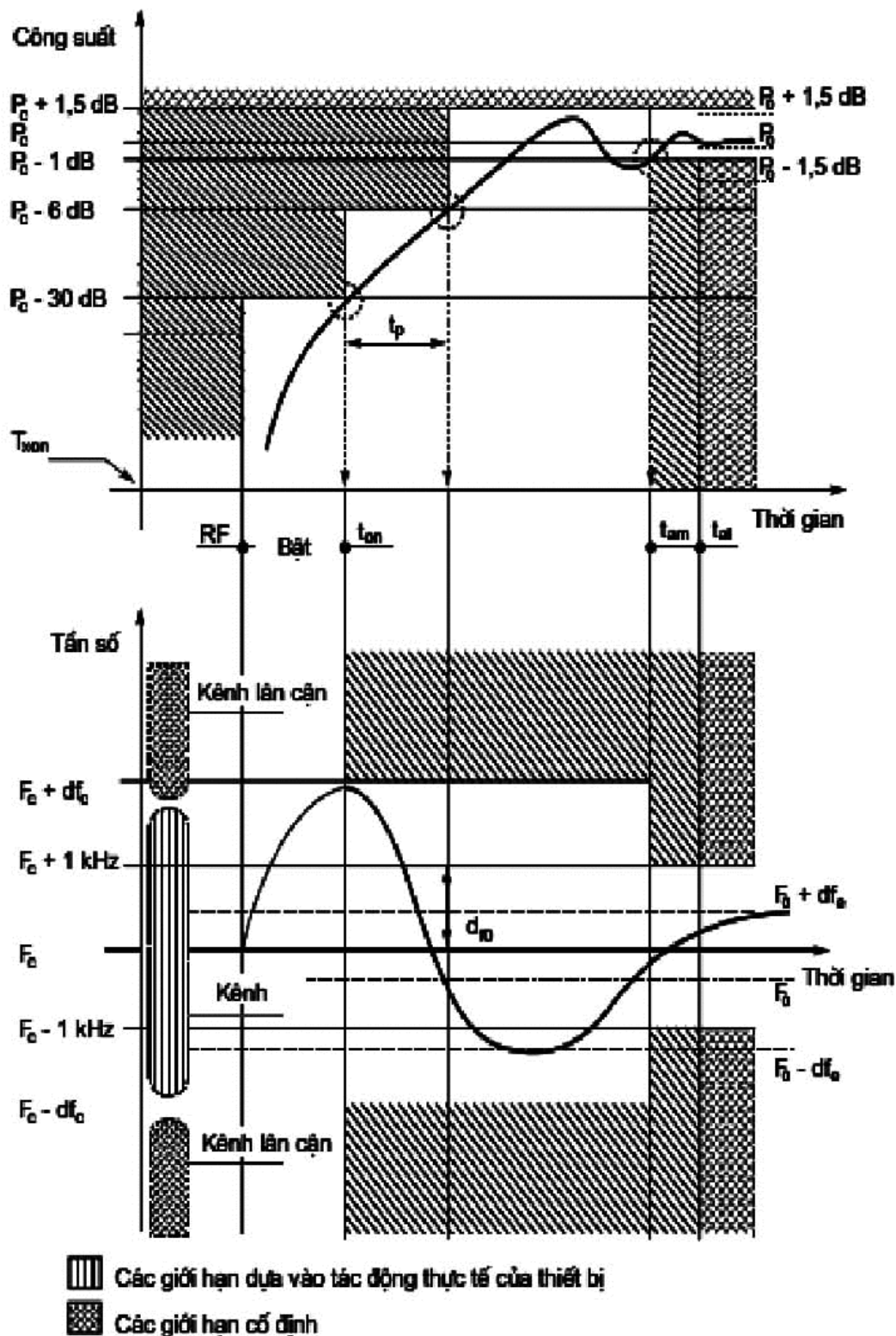
Hình 9 - Thời gian kích hoạt máy phát và tác động quá độ khi bật máy
