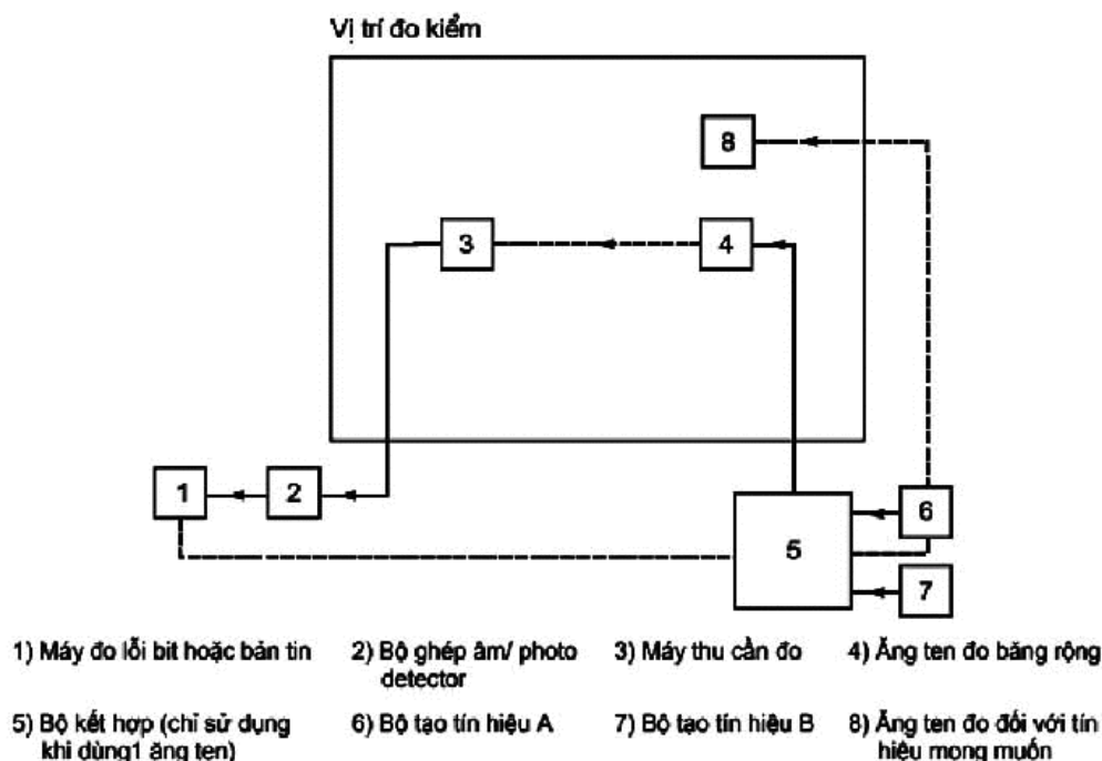
Hình 24 - Sơ đồ đo triết đáp ứng giả
