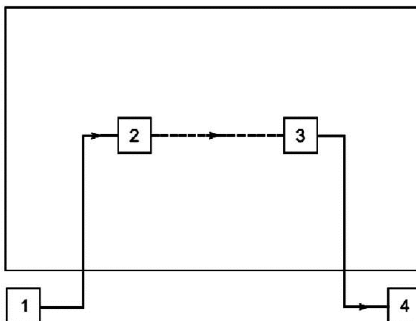
Hình 7 - Sơ đồ đo phát xạ giả bức xạ dùng ăng ten thay thế
