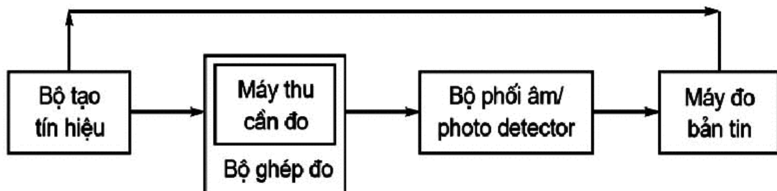
Hình 17 - Sơ đồ đo độ nhạy với bản tin ở điều kiện đo tới hạn
