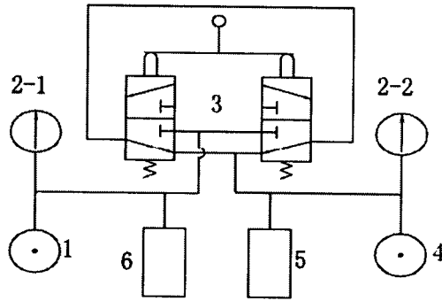
Hình 36: Sơ đồ nguyên lý thử nghiệm an toàn của van khí bị đội áp suất trở lại trở lại của van đổi hướng
