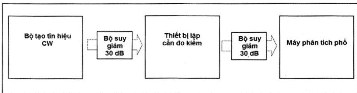
Hình C.2 - Sơ đồ đo tăng ích ngoài băng
