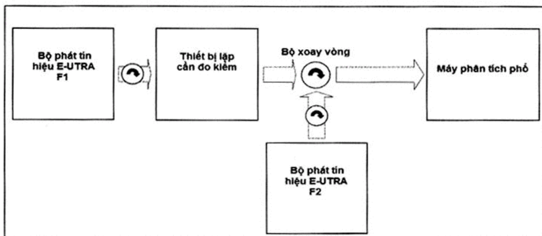
Hình C.6. Sơ đồ đo xuyên điều chế đầu ra
