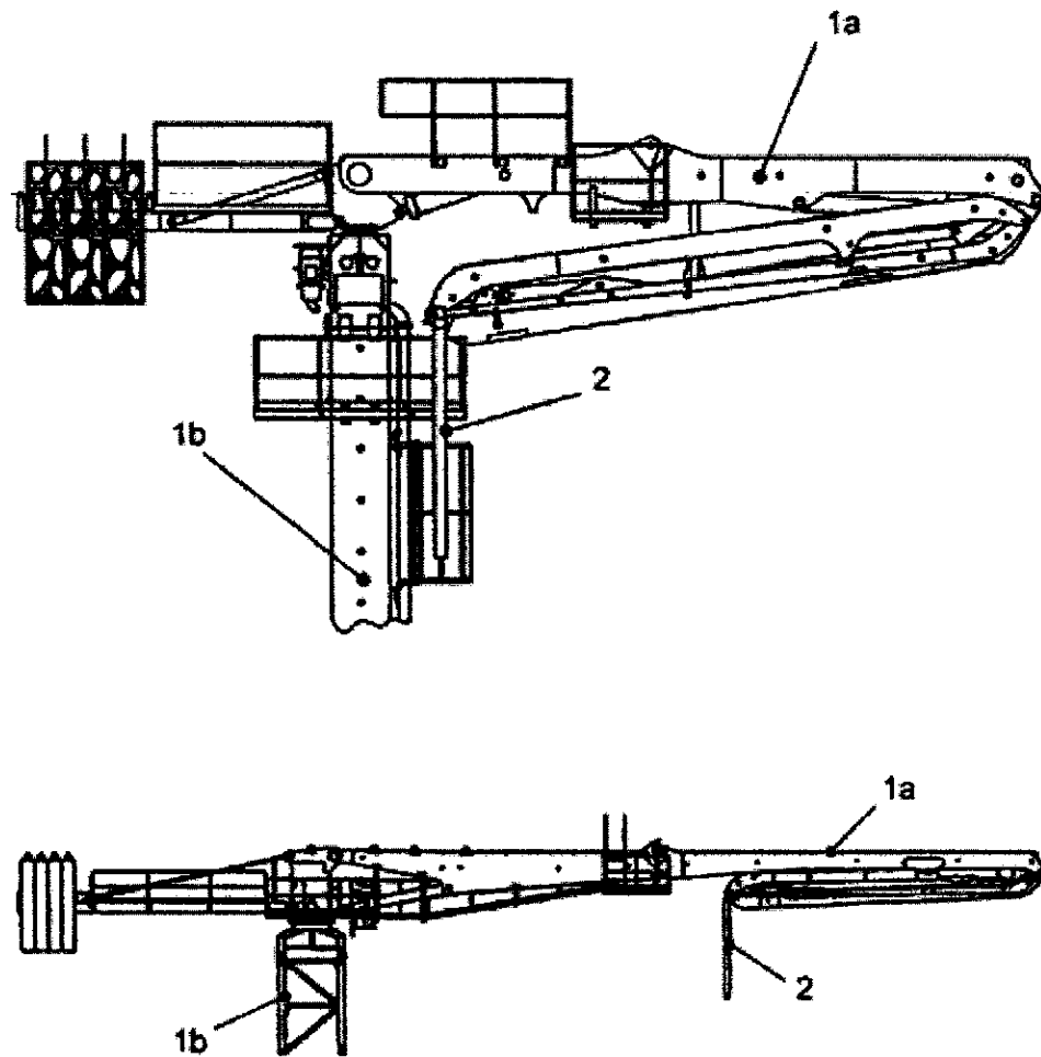
Hình A.1 Cần phân phối bê tông độc lập: 1a – các đoạn cần phân phối bê tông, 1b – trụ đứng, 2 - ống mềm đổ bê tông.
