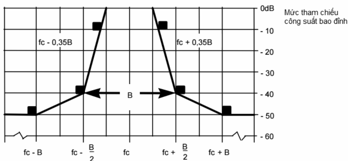
Hình 4. Mặt nạ phổ tần số cho hệ thống điều chế số có B = 600 kHz, 1 200 kHz
