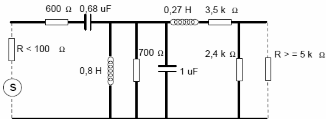
Hình 2. Bộ lọc thụ động
