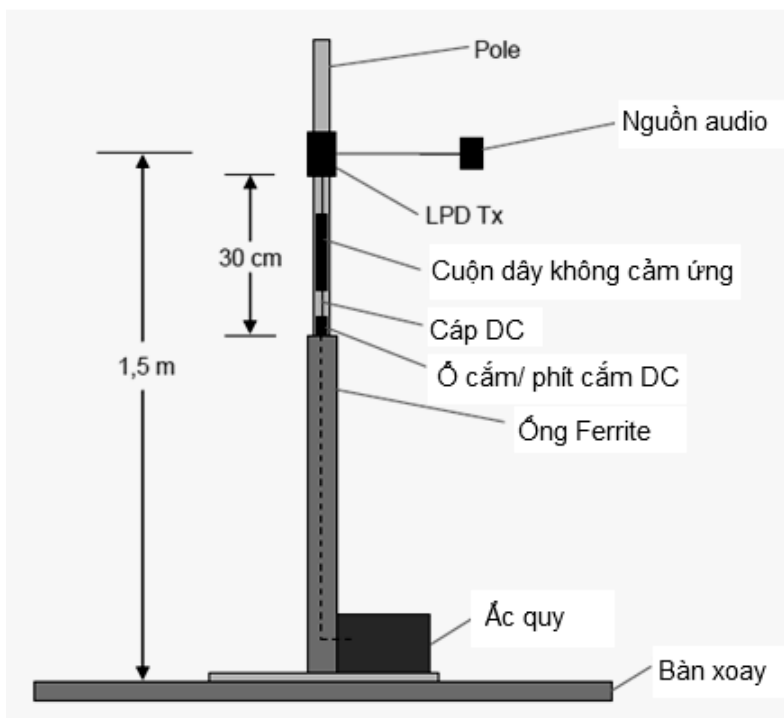
Hình F.1. Bố trí phép đo điển hình đối với thiết bị công suất thấp băng tần II
