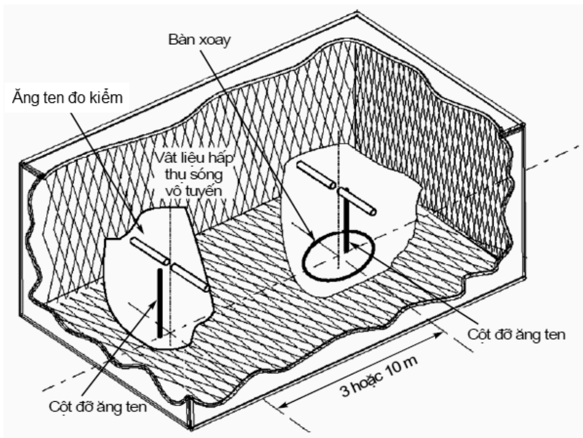
Hình A.1. Buồng triệt phản xạ
