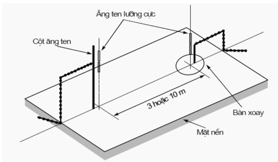
Hình A.3. Vị trí đo kiểm ngoài trời
