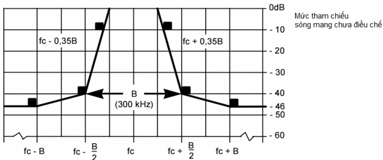
Hình 3. Mặt nạ phổ tần số cho hệ thống điều chế tương tự hoặc điều chế số có B = 300 kHz
