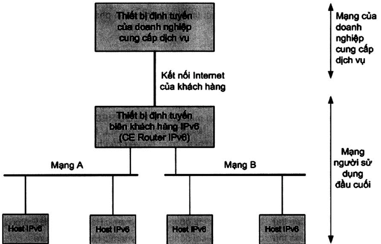
Hình 1 - Mô hình mạng người sử dụng đầu cuối điển hình
