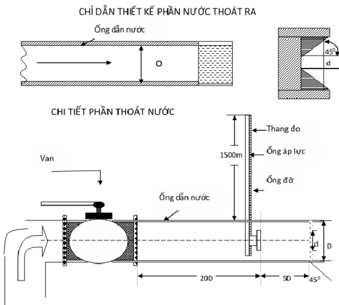
Hình 1-PL. Dụng cụ đo áp lực dùng để xác định lưu lượng khi bơm nước
