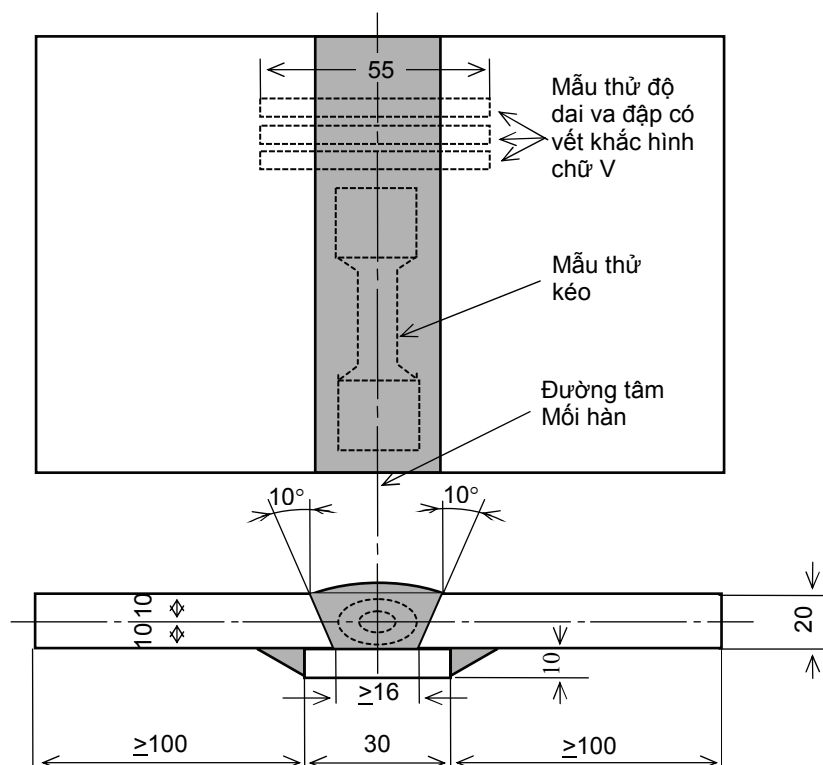
Hình 11. Mẫu thử kim loại đắp (đơn vị: mm)
