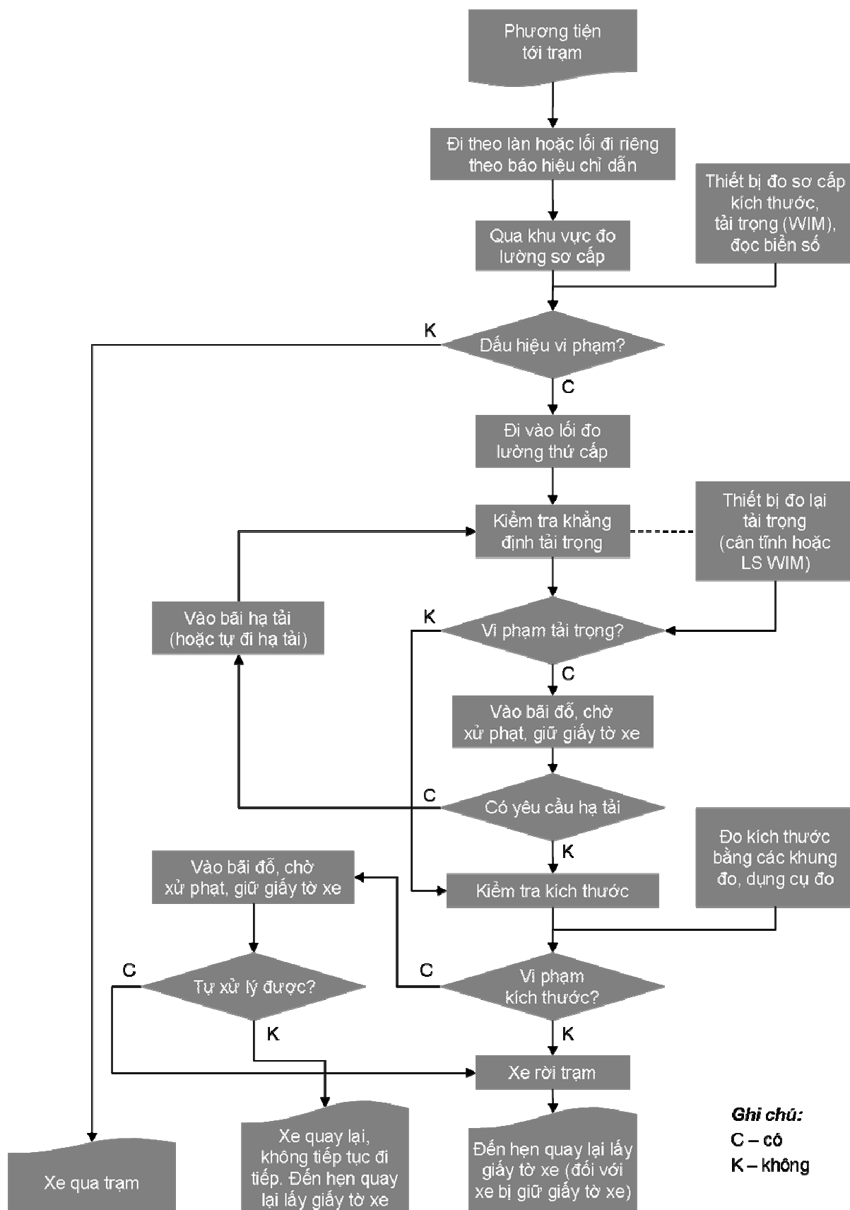
Hình 1. Lưu đồ cơ bản về quy trình kiểm tra và xử lý xe vi phạm tại trạm KTTTX cố định
