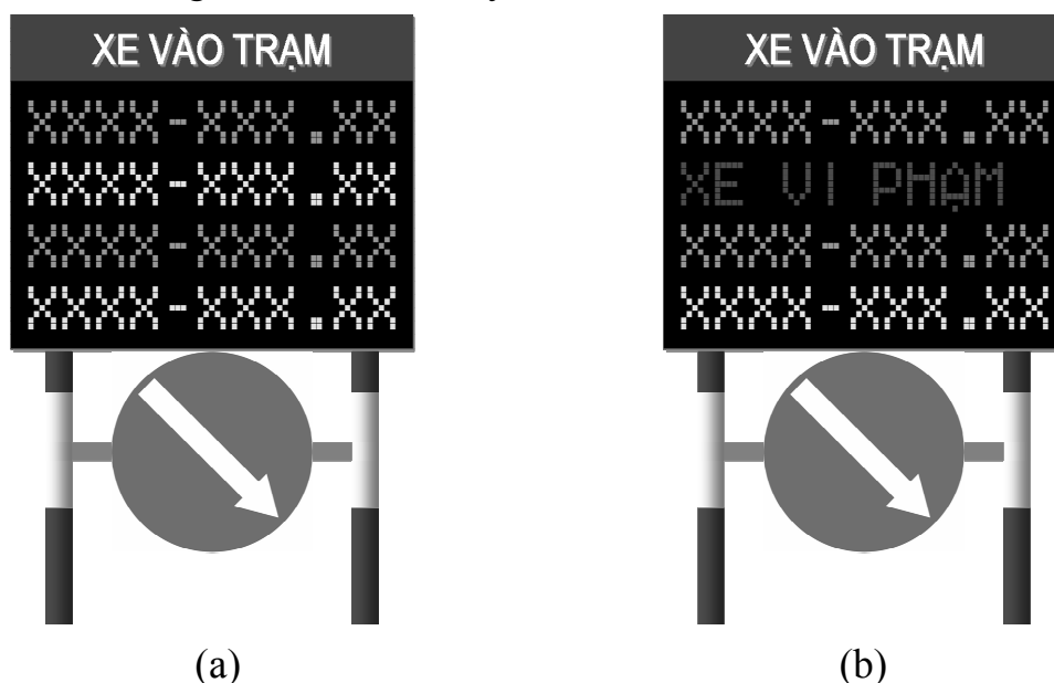
Hình 12. Tổ hợp biển báo đặt tại đầu đảo tách lối xe vi phạm vào trạm (XXXX-XXX.XX là biển số xe)
