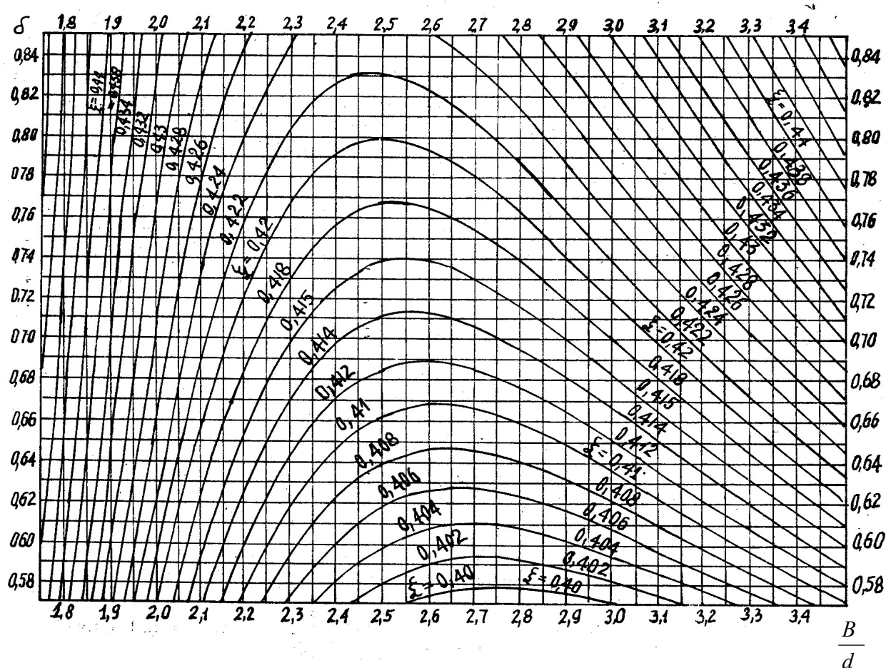
Hình 5. Xác định hệ số \xi
