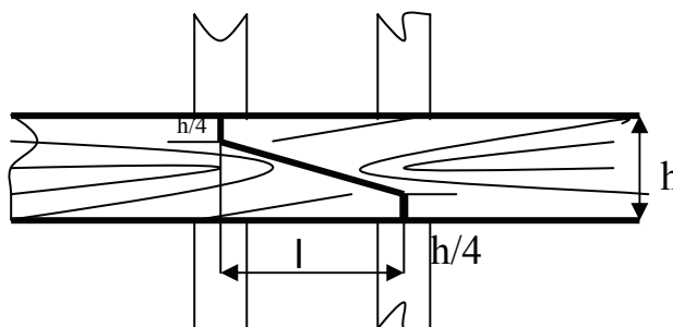
Hình 4. Quy cách mỗi nổi gài
