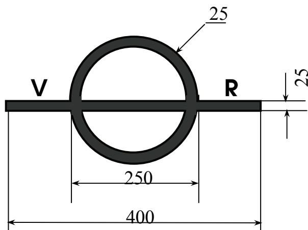
Hình 6. Dấu mạn khô
